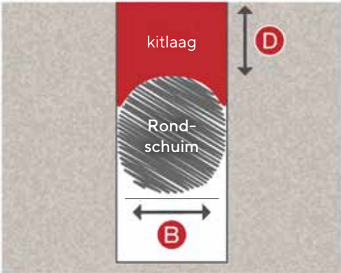
B= Voegbreedte D= Voegdiepte
